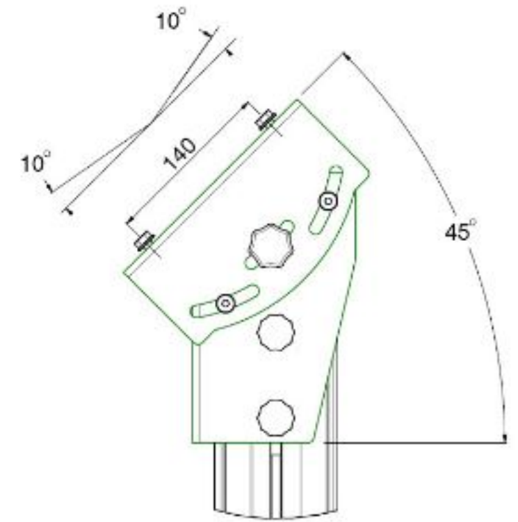
DETAIL B SCALE 0.150
