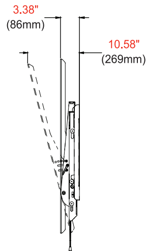
SEITENANSICHT +15°/-5° NEIGUNG
